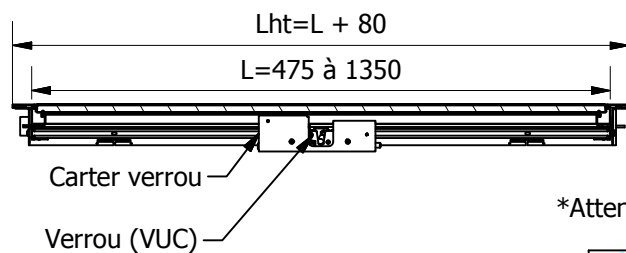
A-A ( 1/16 )
